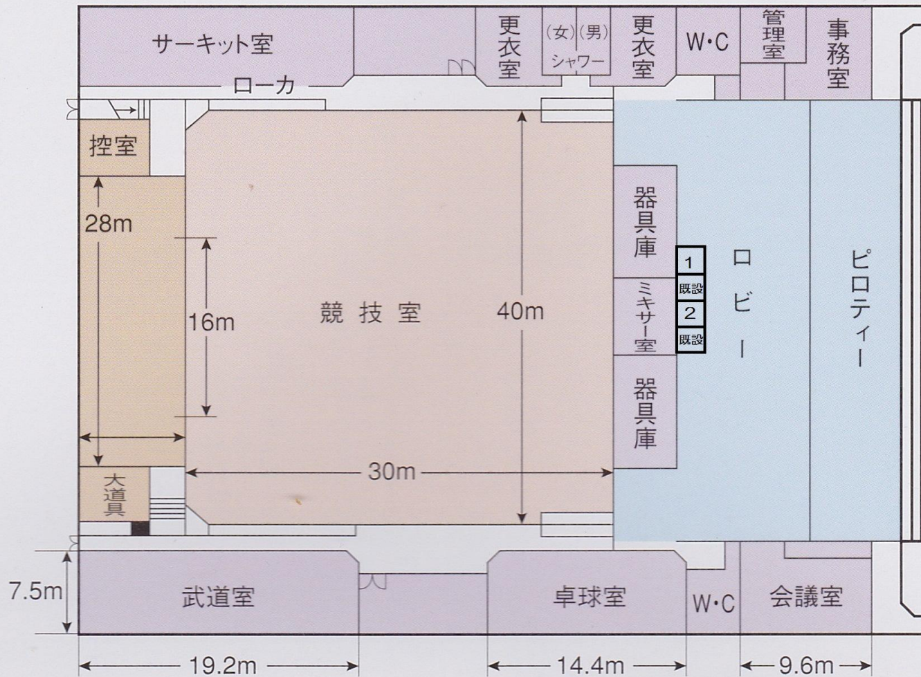
1階平面図
