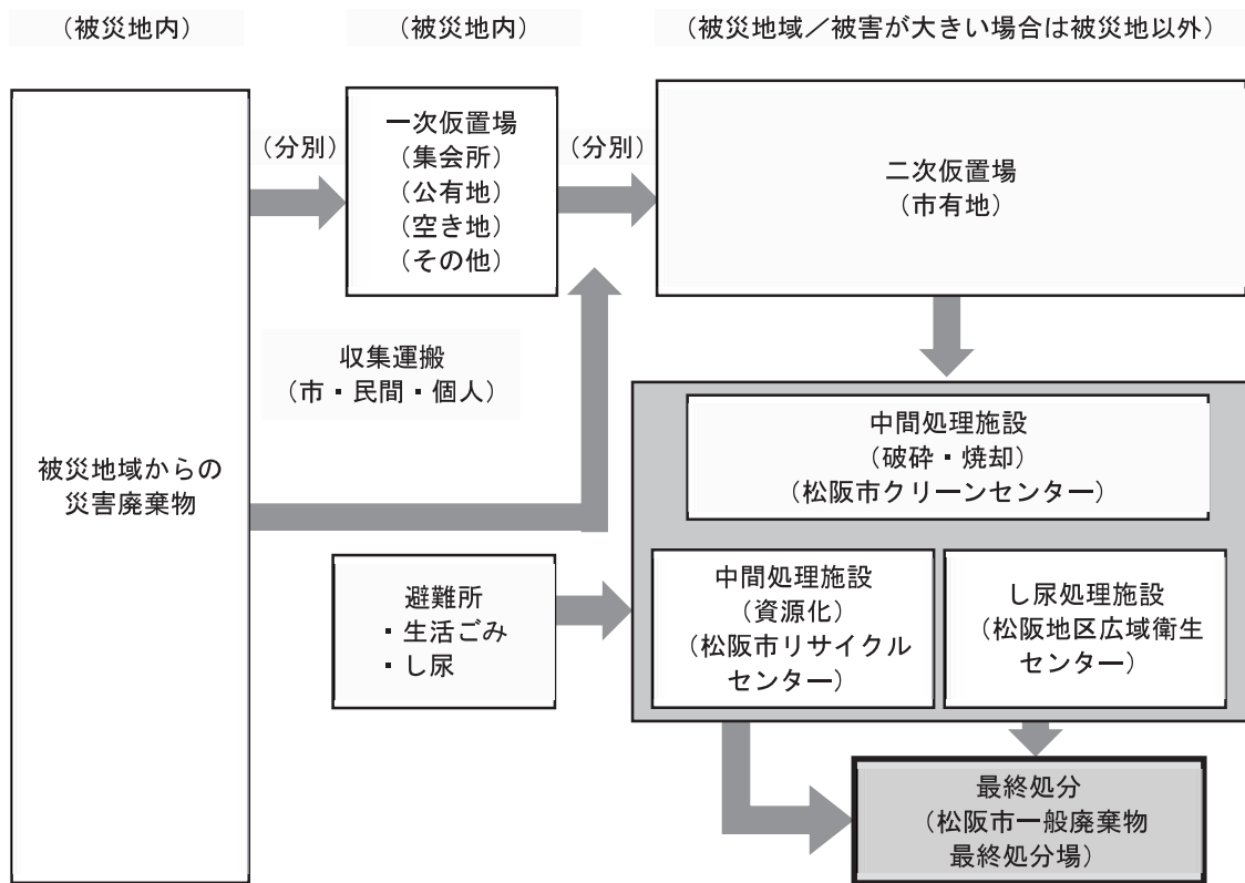
災害廃棄物処理フロー
