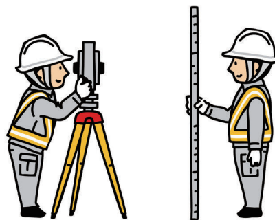
▲地籍調査
