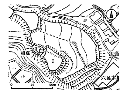
図2「縄張り図」
