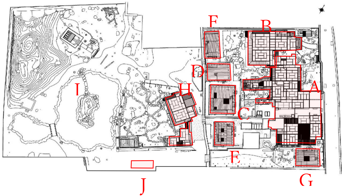
旧長谷川治郎兵衛家 平面図
