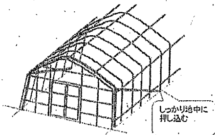
妻面補強の参考例 (風対策に有効)
