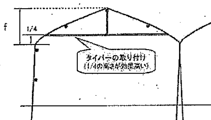
タイバーによる肩部の補強事例
