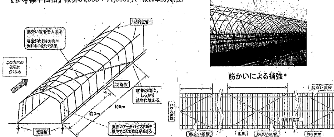
筋交いによる妻面の補強方法事例
