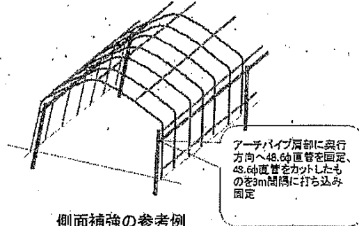
側面補強の参考例
