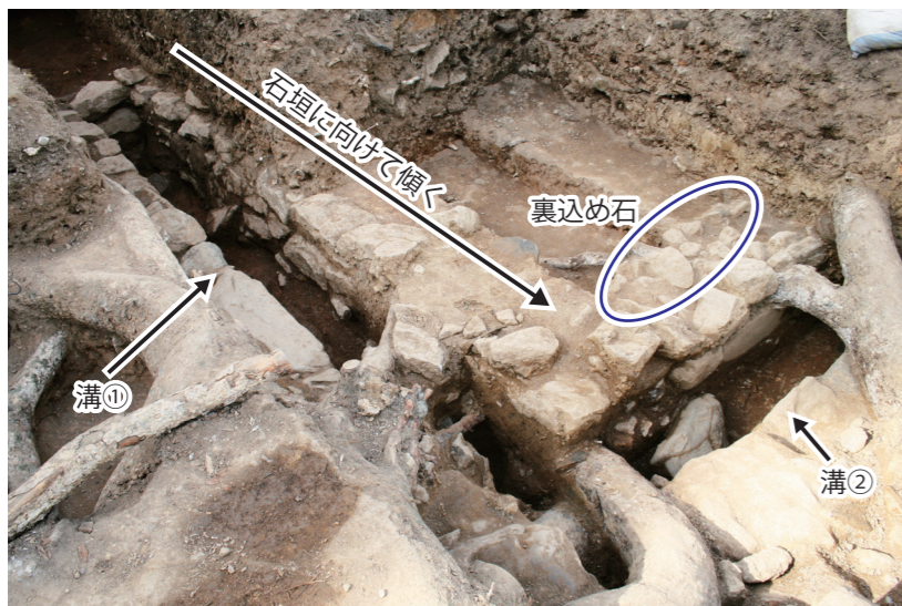
写真2 石組み溝
