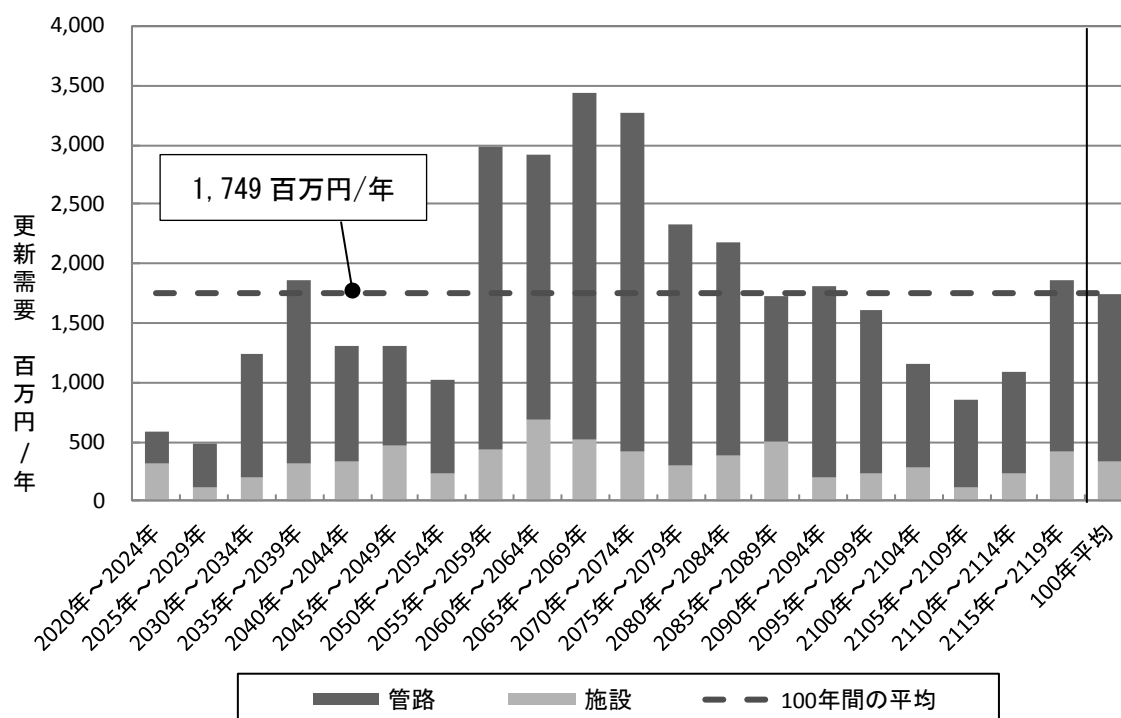
図 3.2.1 更新需要の見通し（更新基準年数で更新した場合）
