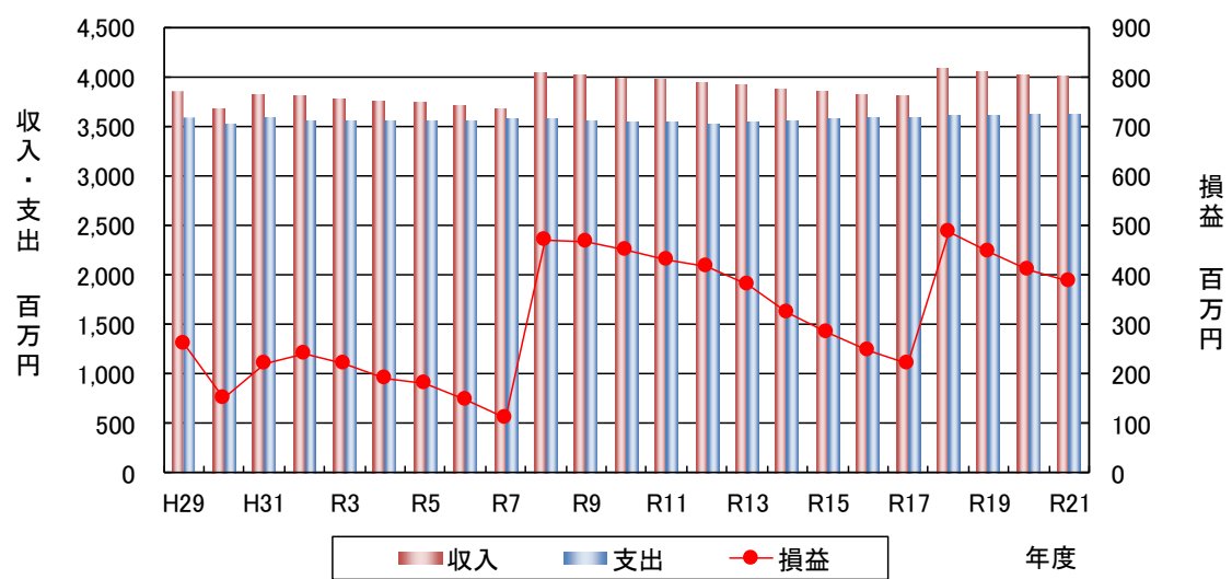
図 4.2.3 収益的収支（ケース 4）
