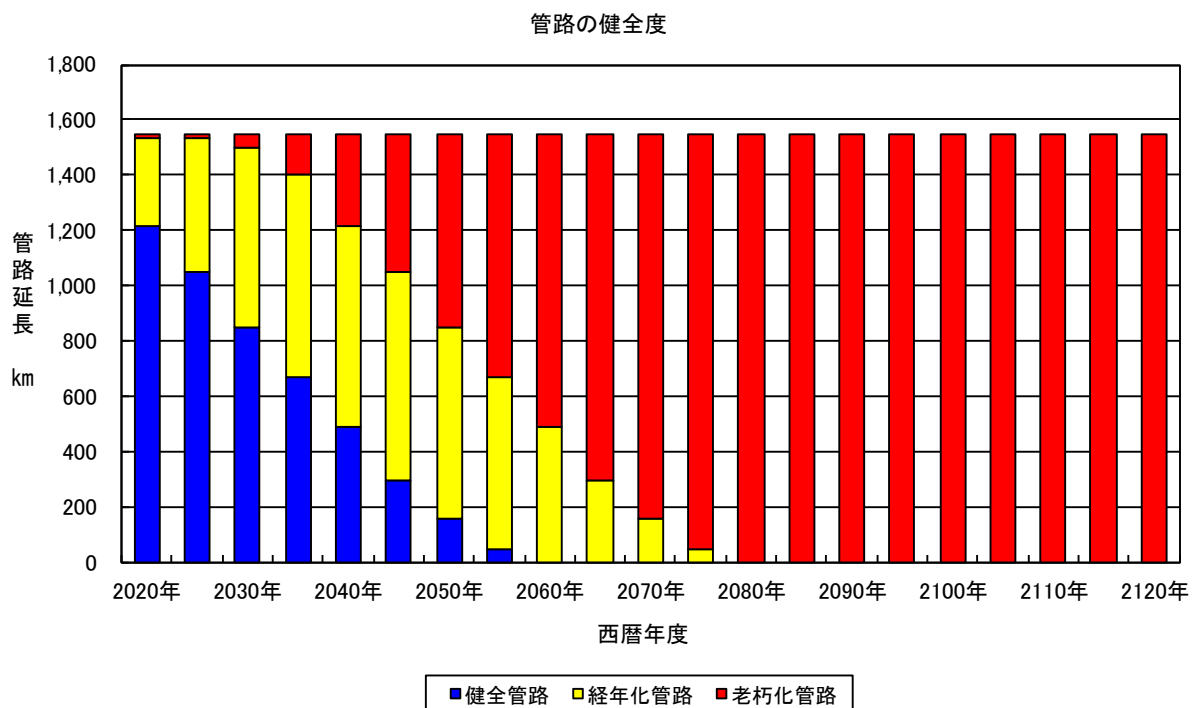
図 2.2.2 管路の健全度（更新を行わなかった場合）
