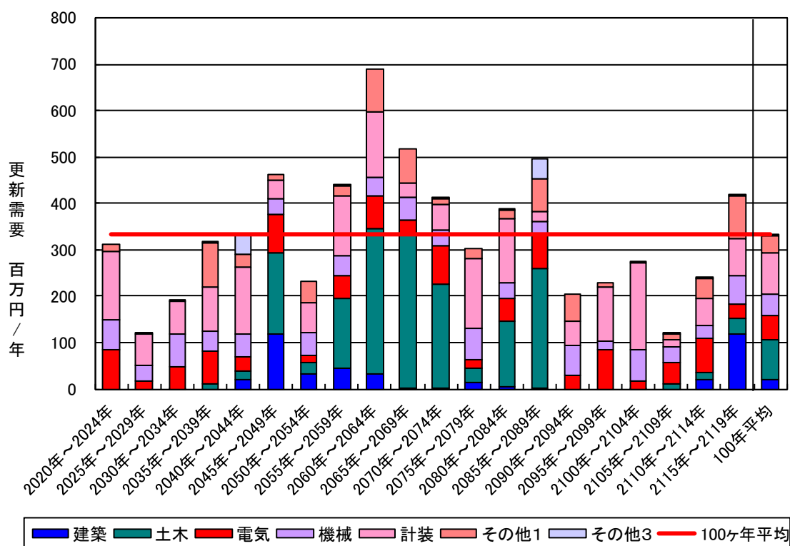
図 3.2.2 施設の更新需要（更新基準年数で更新した場合）
