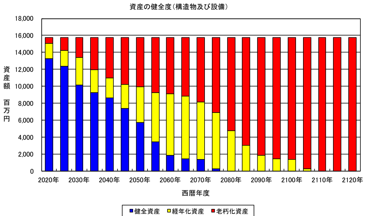
図 2.2.1 構造物及び設備の健全度（更新を行わなかった場合）
