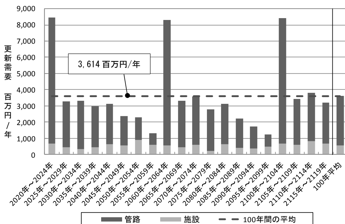
図 2.2.3 更新需要の見通し（法定耐用年数で更新した場合）
