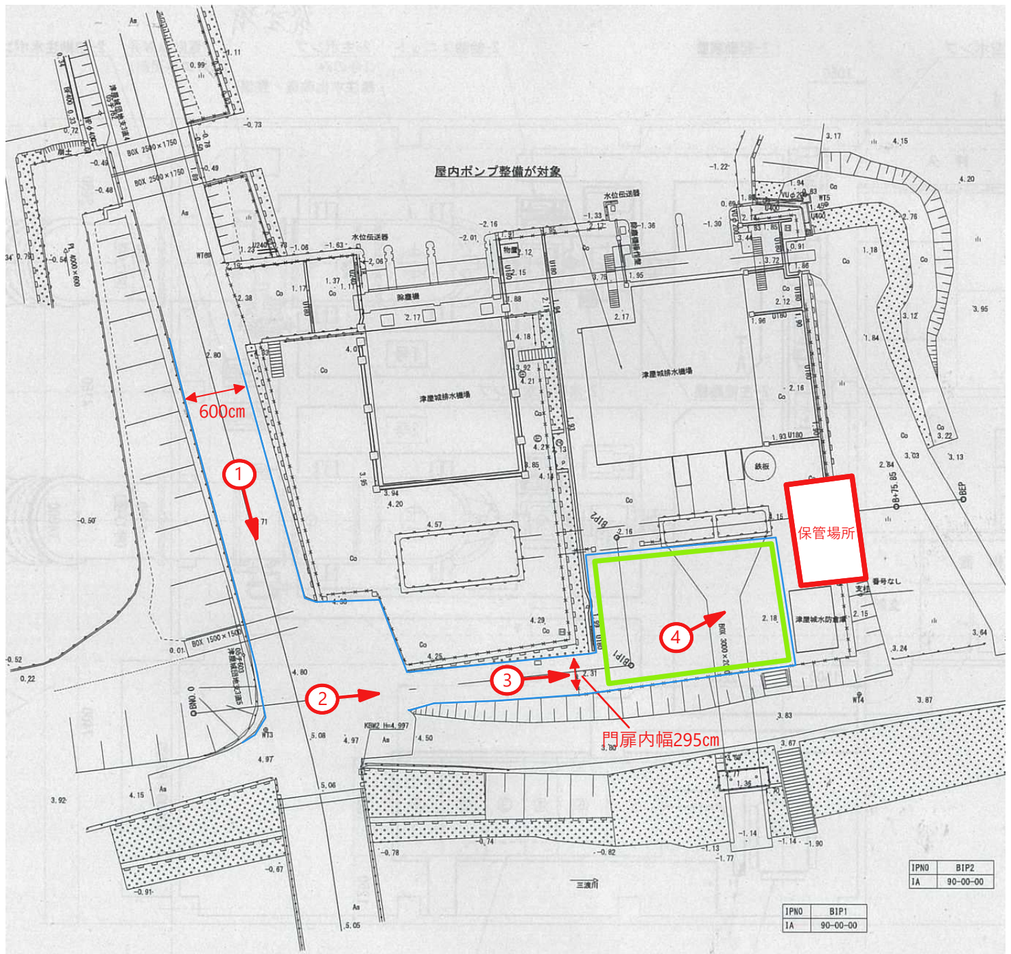
場内平面図
