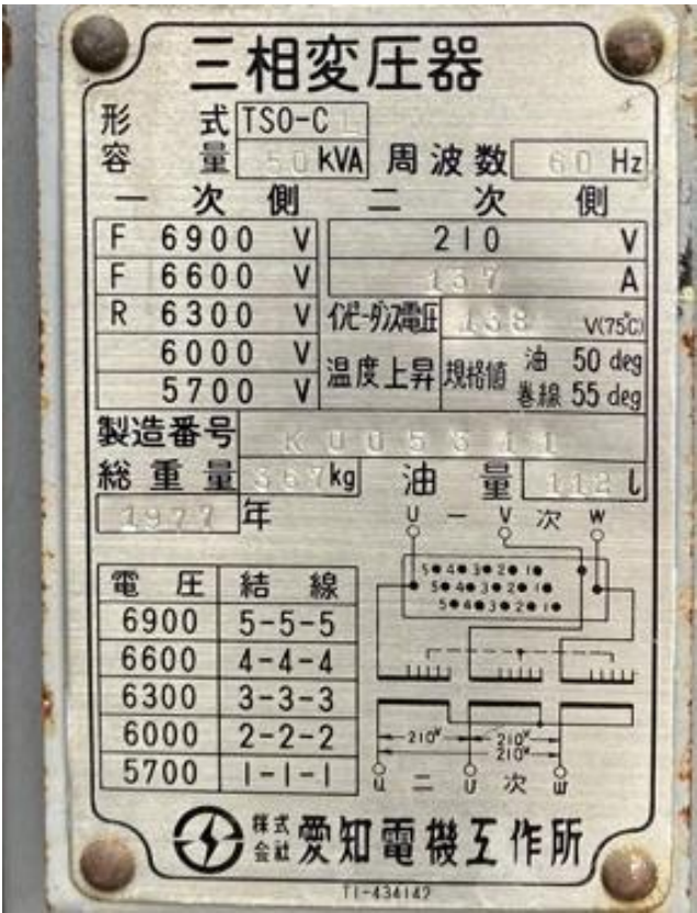
写真2.変圧器「TSO-CL」銘板 ※製造番号：K005311
