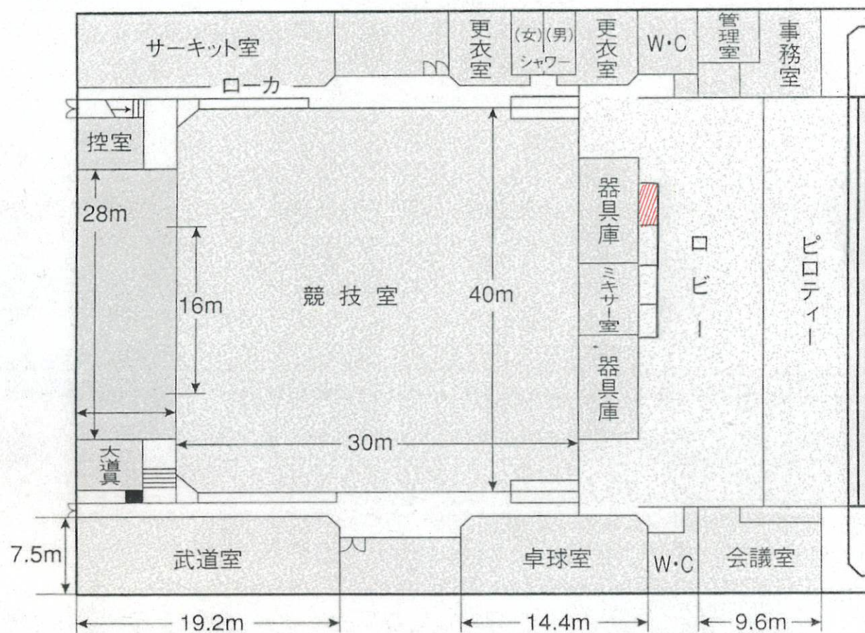
1 階平面図
