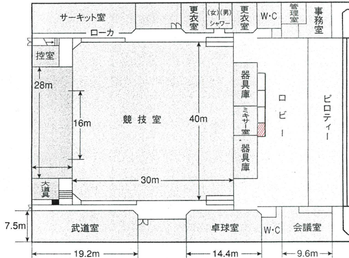
1 階平面図
