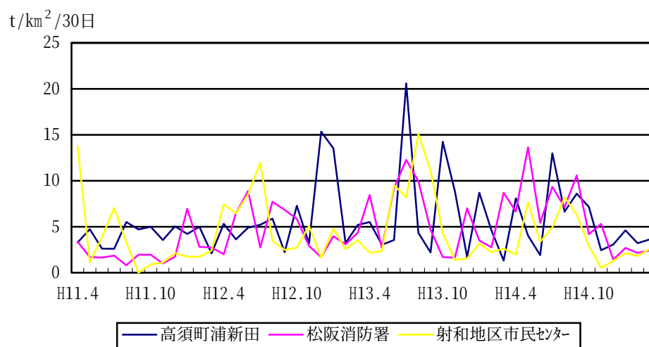
図 3-1-7 平成 11 年度～14 年度の降下ばいじんの経年変化
