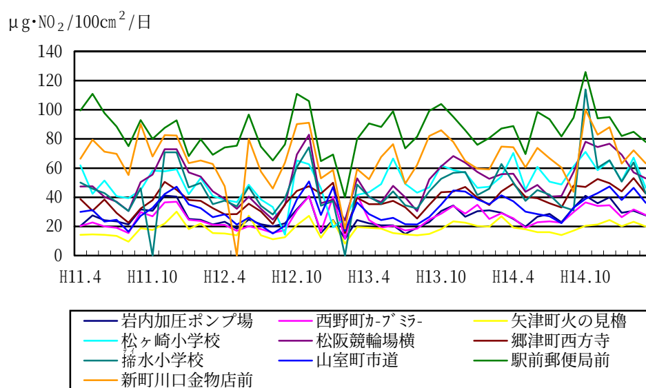
図 3-1-6 平成 11 年度～14 年度の二酸化窒素（TEA プレート法）の経年変化
