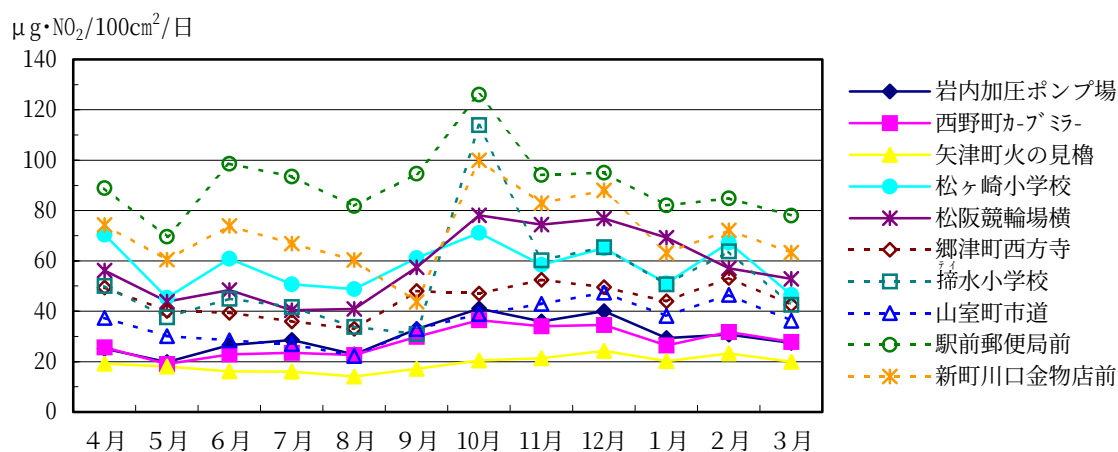
図 3-1-2 二酸化窒素の経月変化
