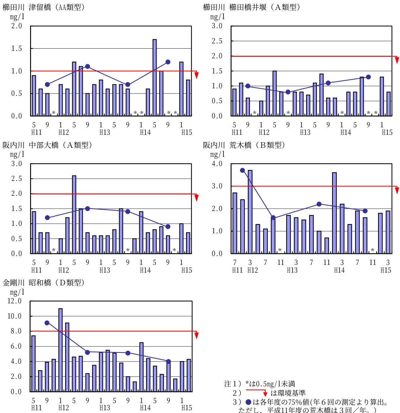
図 3-2-1 河川に係る環境基準点 5 地点における平成 11 年度～14 年度の BOD の経年変化
