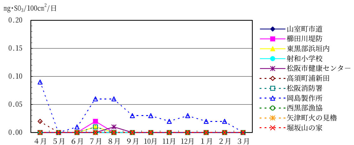
図 3-1-1 硫黄酸化物の経月変化
