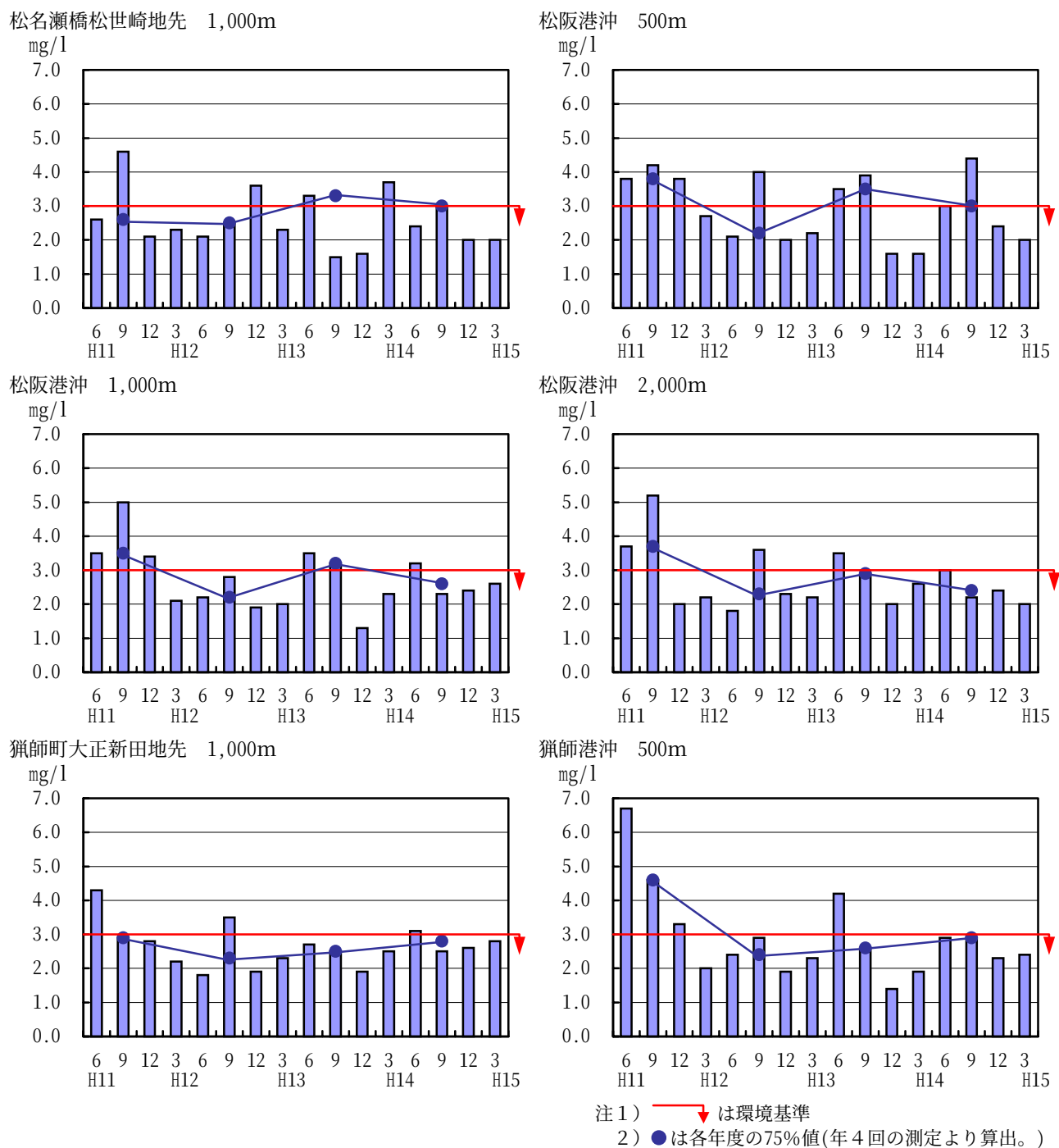
図3-2-2 海域に係る平成11年度～14年度のCODの経年変化
