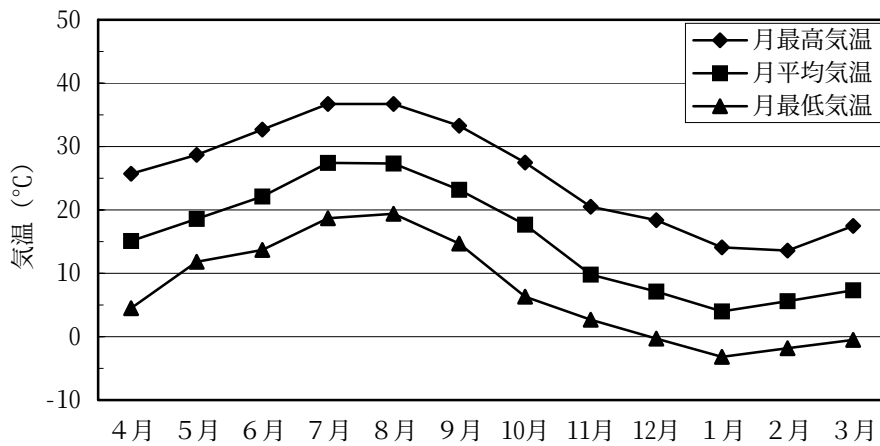
図 1-3 平成 14 年度の月平均気温、月最高・最低気温
