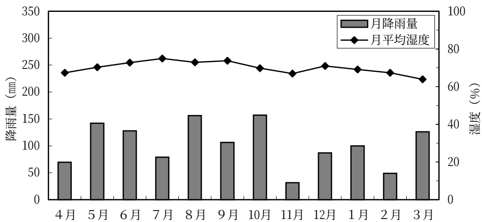
図 1-4 平成 14 年度の月別降雨量と月平均湿度
