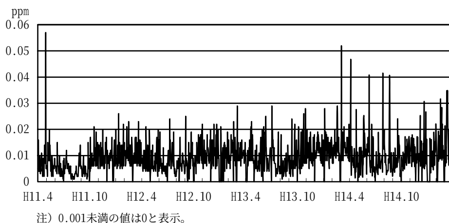
図3-1-4(2) 平成11年度～14年度の二酸化硫黄日平均値の経年変化(2) ー高須町浦新田ー
