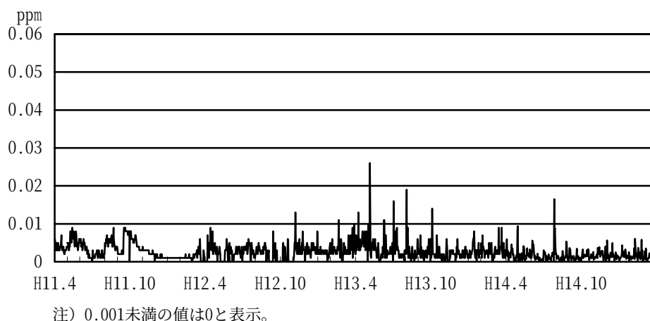
図3-1-4(1) 平成11年度～14年度の二酸化硫黄日平均値の経年変化(1) ー松阪市健康センターー
