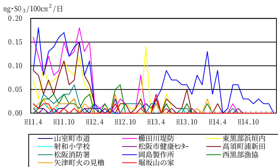
図 3-1-5 平成 11 年度～14 年度の硫黄酸化物（二酸化鉛法）の経年変化
