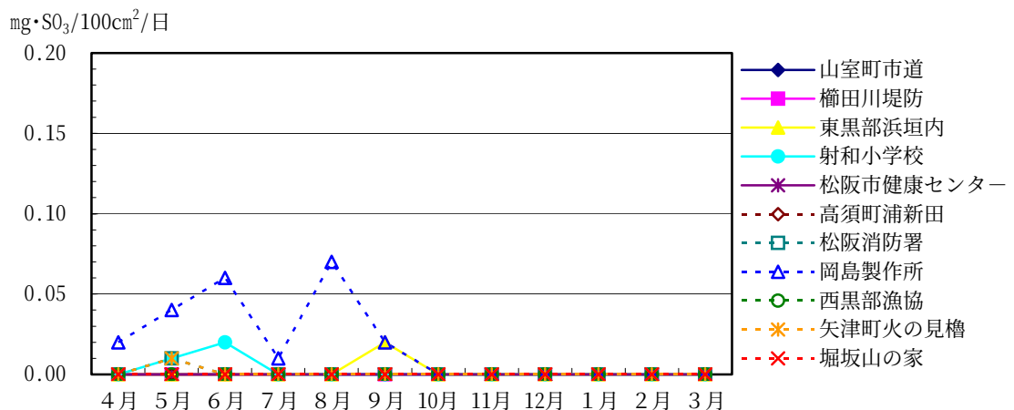
図 3-1-1 硫黄酸化物の経月変化
