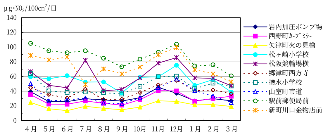
図 3-1-2 二酸化窒素の経月変化
