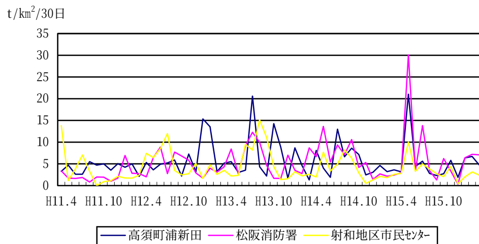
図3-1-7 平成 11 年度～15 年度の降下ばいじんの経年変化
