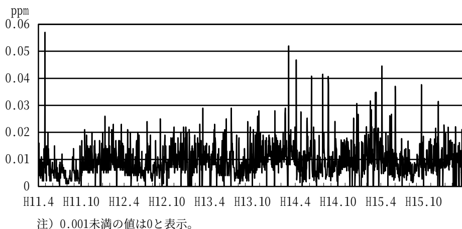
図3-1-4(2) 平成11年度～15年度の二酸化硫黄日平均値の経年変化(2) ー高須町浦新田ー
