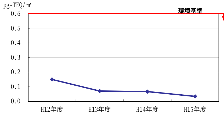
図3-6-1 ダイオキシン類（コプラナーPCBを含む）の経年変化 ー大気質ー
