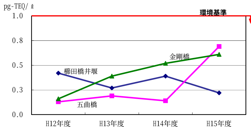
図3-6-2 ダイオキシン類（コプラナーPCBを含む）の経年変化 ー水質ー
