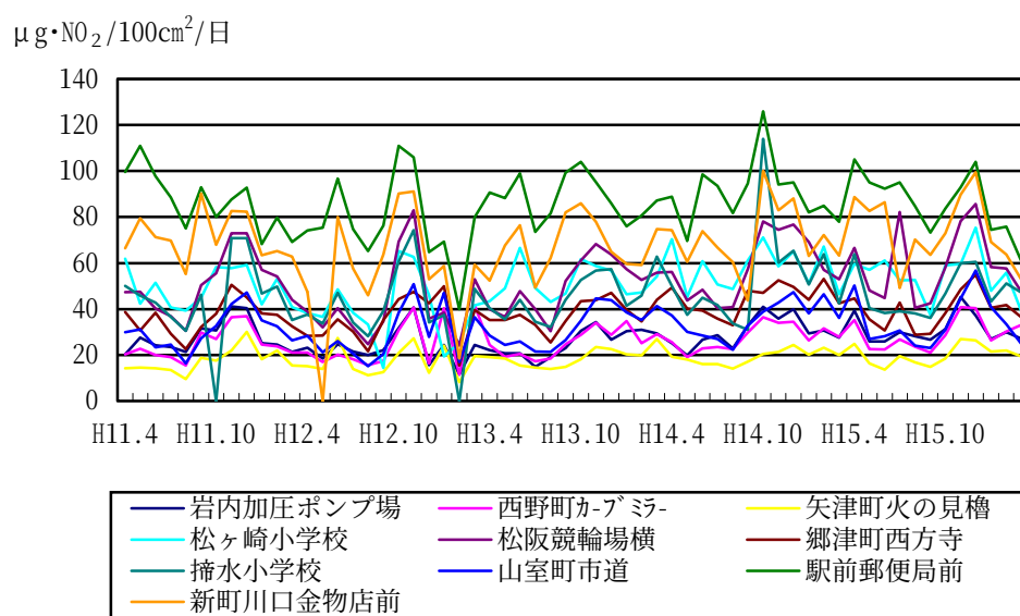
図 3-1-6 平成 11 年度～15 年度の二酸化窒素（TEA プレート法）の経年変化
