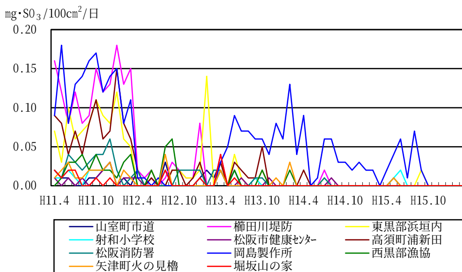
図 3-1-5 平成 11 年度～15 年度の硫黄酸化物（二酸化鉛法）の経年変化
