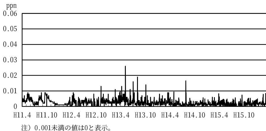
図3-1-4(1) 平成11年度～15年度の二酸化硫黄日平均値の経年変化(1) ー松阪市健康センターー
