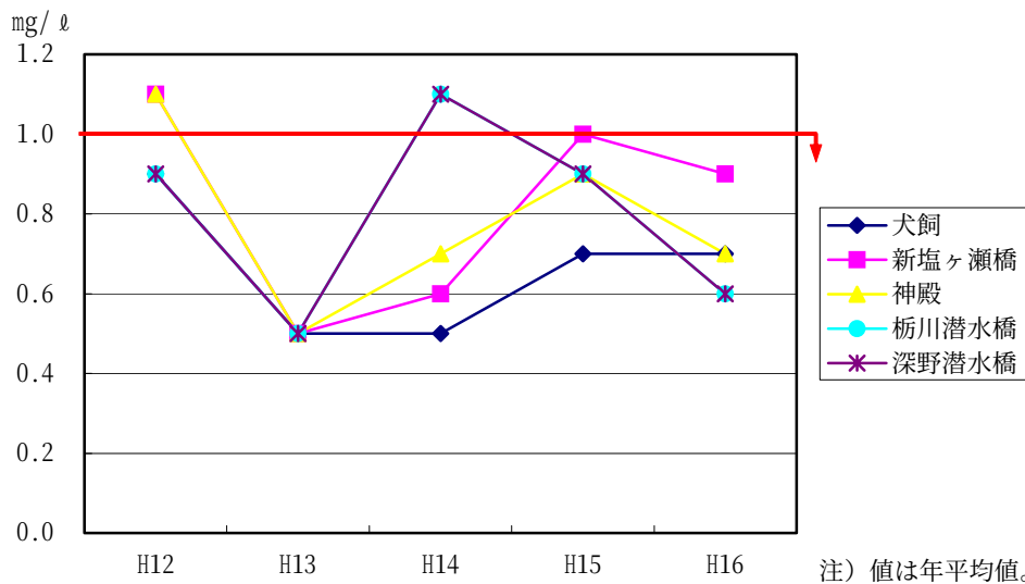
図 3-2-1 飯南管内及び飯高管内河川調査地点における平成 12 年度～16 年度の BOD の経年変化
