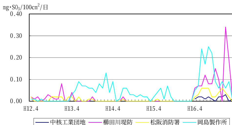
図 3-1-5 平成 12 年度～16 年度の硫黄酸化物（二酸化鉛法）の経年変化
