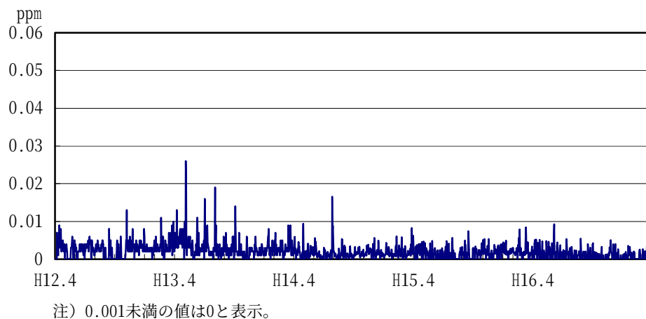
図3－1－4(1) 平成12年度～16年度の二酸化硫黄日平均値の経年変化 －松阪市健康センター－
