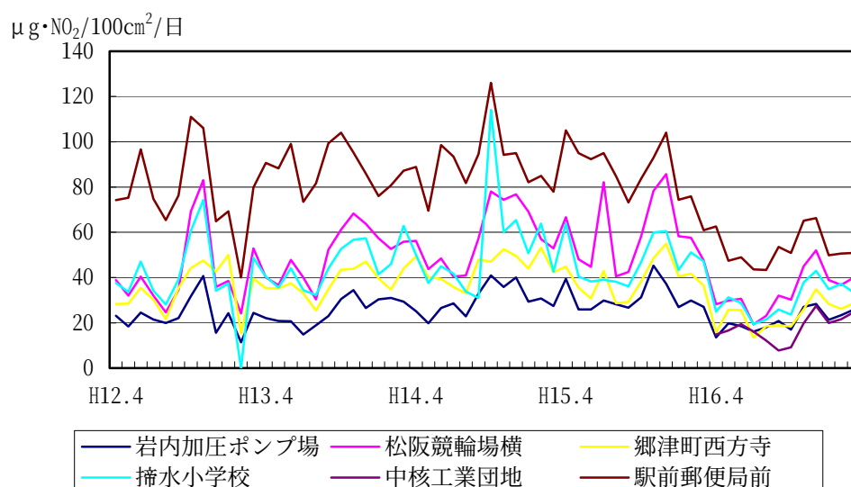
図 3-1-6 平成 12 年度～16 年度の二酸化窒素（TEA プレート法）の経年変化
