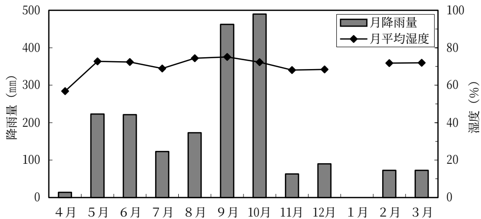
図1-4 平成16年度の月別降雨量と月平均湿度
