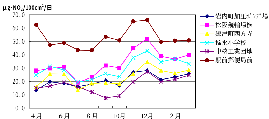
図3-1-2 二酸化窒素の経月変化
