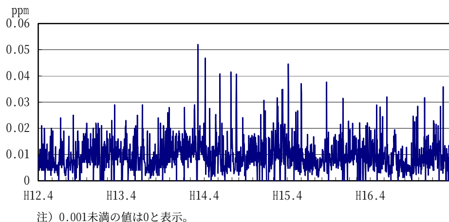
図3－1－4(2) 平成12年度～16年度の二酸化硫黄日平均値の経年変化 －高須町浦新田－
