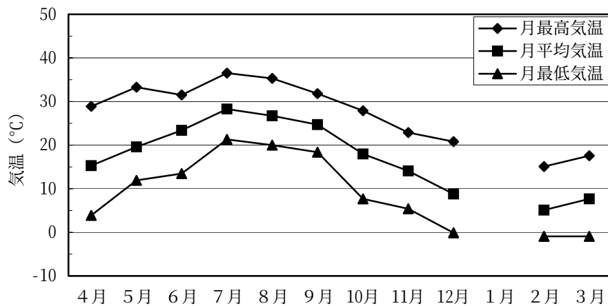
図1-3 平成16年度の月平均気温、月最高・最低気温
