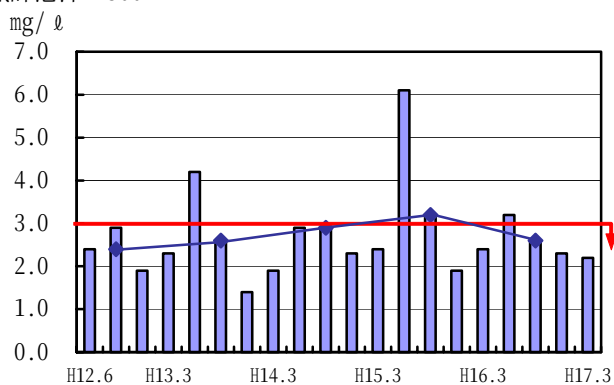
図3-2-2 海域に係る平成12年度～16年度のCODの経年変化
