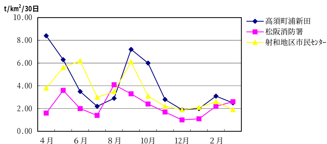
図3-1-3 降下ばいじんの経月変化
