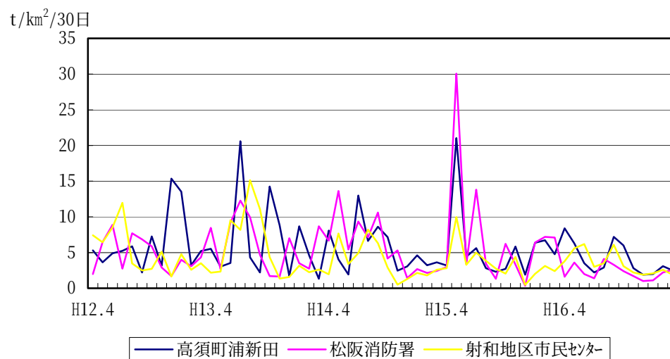
図 3-1-7 平成 12 年度～16 年度の降下ばいじんの経年変化
