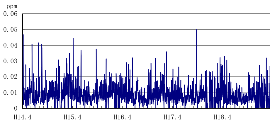
図3-1-4(2) 平成14年度～18年度の二酸化硫黄日平均値の経年変化 —高須町浦新田—
