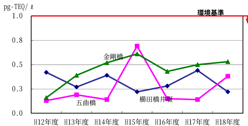
図3-6-2 ダイオキシン類（コプラナーPCBを含む）の経年変化 ー水質ー
