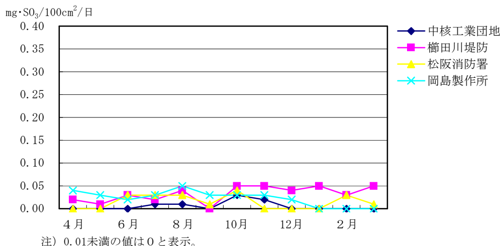
図 3-1-1 硫黄酸化物の経月変化
