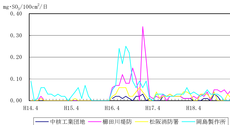
図3-1-5 平成14年度～18年度の硫黄酸化物（二酸化鉛法）の経年変化
