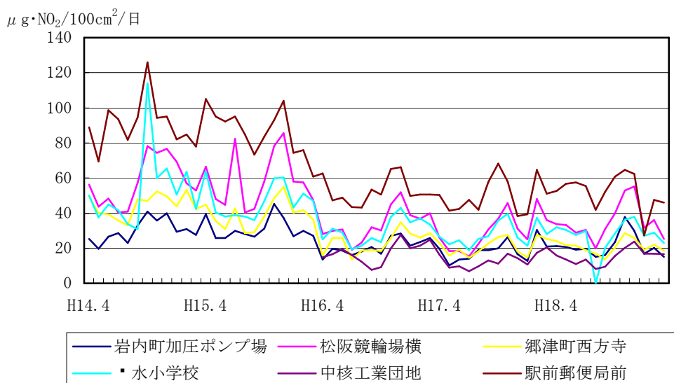
図3-1-6 平成14年度～18年度の二酸化窒素（TEA プレート法）の経年変化
