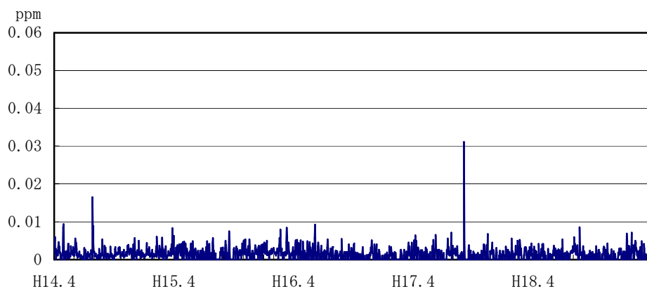
図3-1-4(1) 平成14年度～18年度の二酸化硫黄日平均値の経年変化 —松阪市健康センター—
