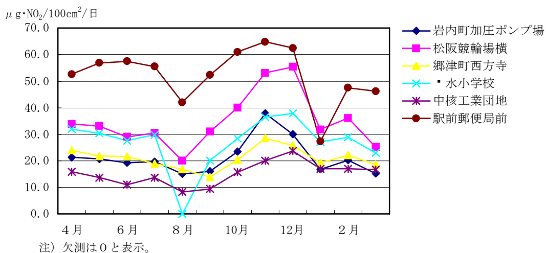
図3-1-2 二酸化窒素の経月変化
