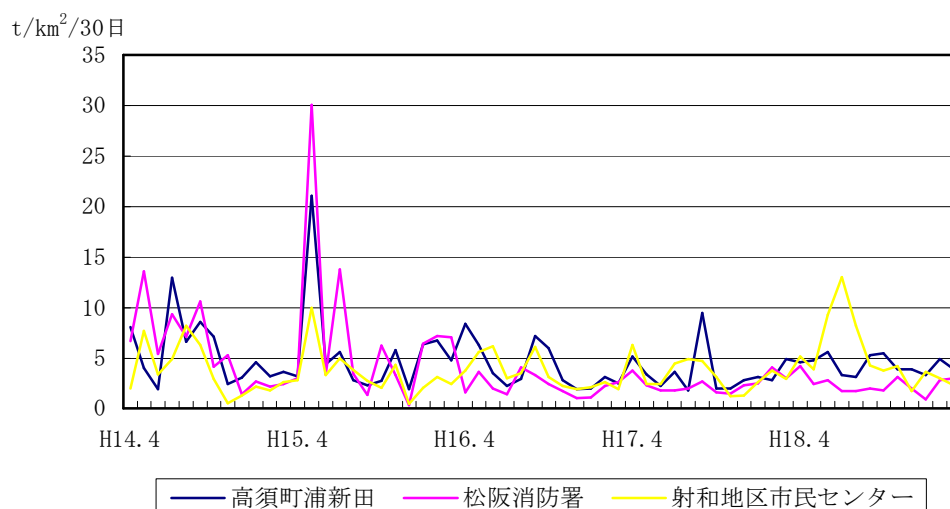
図3-1-7 平成14年度～18年度の降下ばいじんの経年変化
