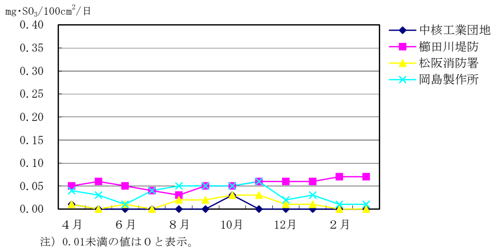
図3-1-1 硫黄酸化物の経月変化
