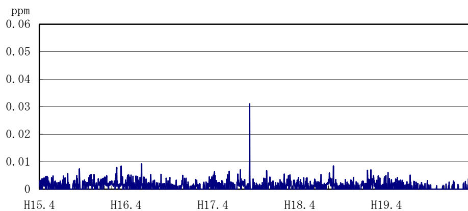
図3-1-4(1) 平成15年度～19年度の二酸化硫黄日平均値の経年変化 ー松阪市健康センターー
