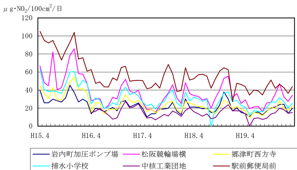
図3-1-6 平成15年度～19年度の二酸化窒素（TEA プレート法）の経年変化
