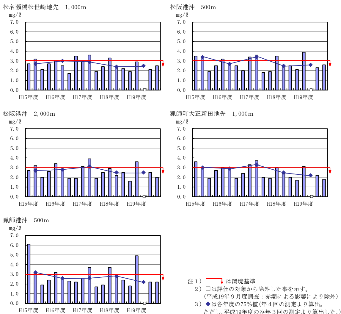
図3-2-2 海域調査地点における平成15年度～19年度のCODの経年変化
