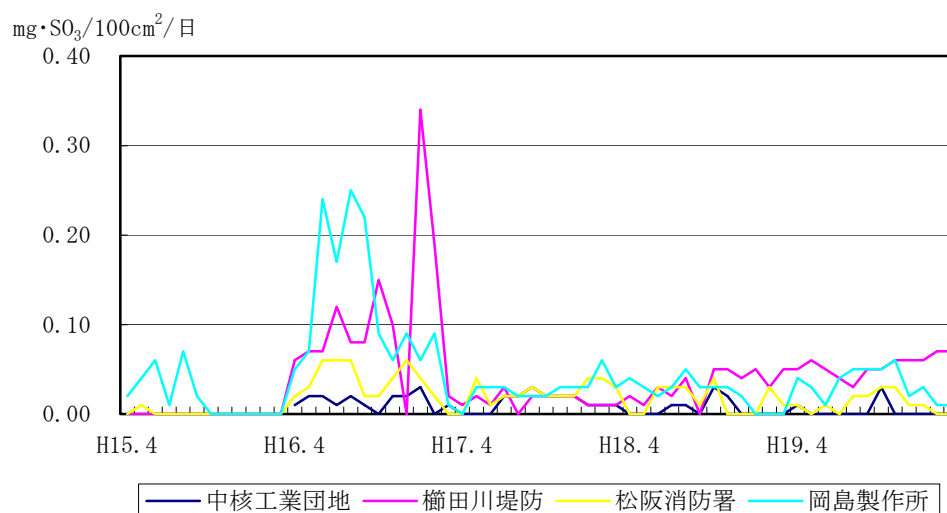
図3-1-5 平成15年度～19年度の硫黄酸化物（二酸化鉛法）の経年変化
