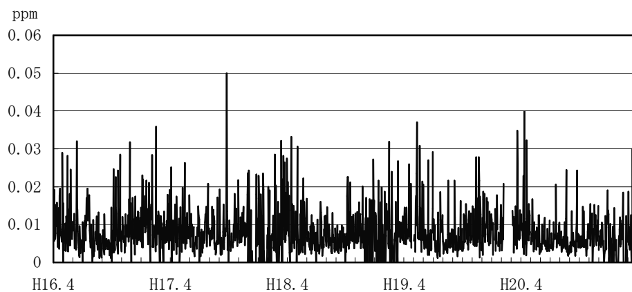
図3-1-2(2) 平成16年度～20年度の二酸化硫黄日平均値の経年変化 —高須町浦新田—
