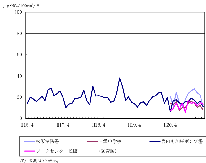
図3-1-3(3) 平成16年度～20年度の二酸化窒素（TEAプレート法）の経年変化
