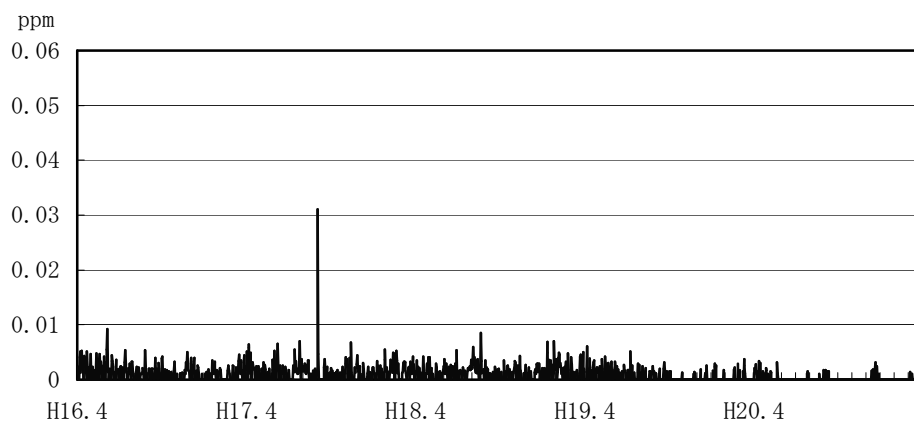
図3-1-2(1) 平成16年度～20年度の二酸化硫黄日平均値の経年変化 —松阪市健康センター—
