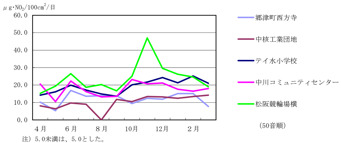
図 3-1-1 (2) 二酸化窒素の経月変化
