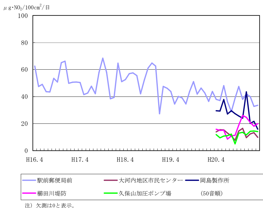
図3-1-3(1) 平成16年度～20年度の二酸化窒素（TEAプレート法）の経年変化
