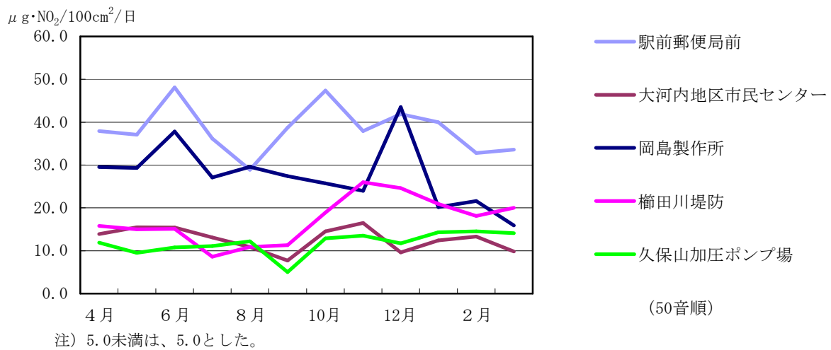
図 3-1-1 (1) 二酸化窒素の経月変化
