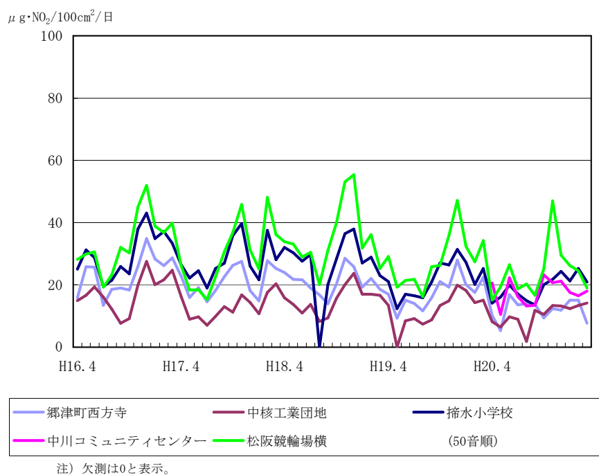
図3-1-3(2) 平成16年度～20年度の二酸化窒素（TEAプレート法）の経年変化
