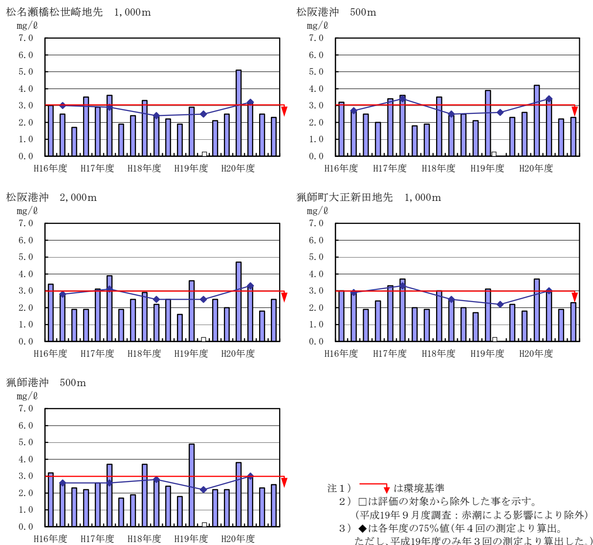
図3-2-2 海域調査地点における平成16年度～20年度のCODの経年変化
