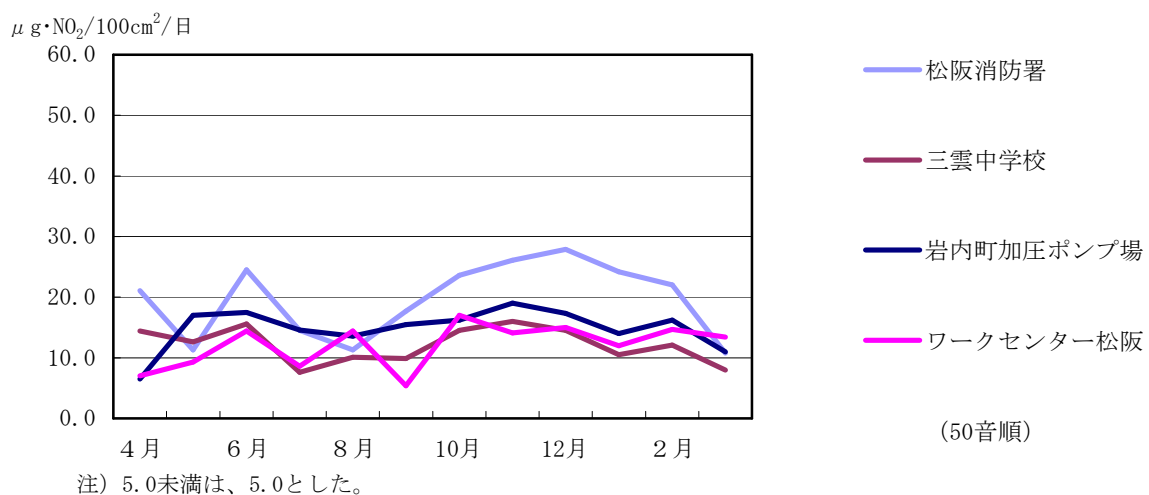
図 3-1-1 (3) 二酸化窒素の経月変化
