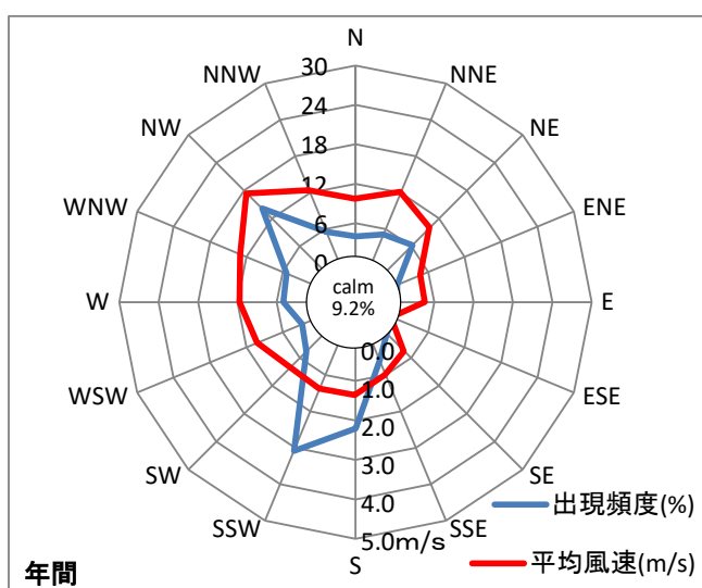
図 7-1-1.2 年間風配図
