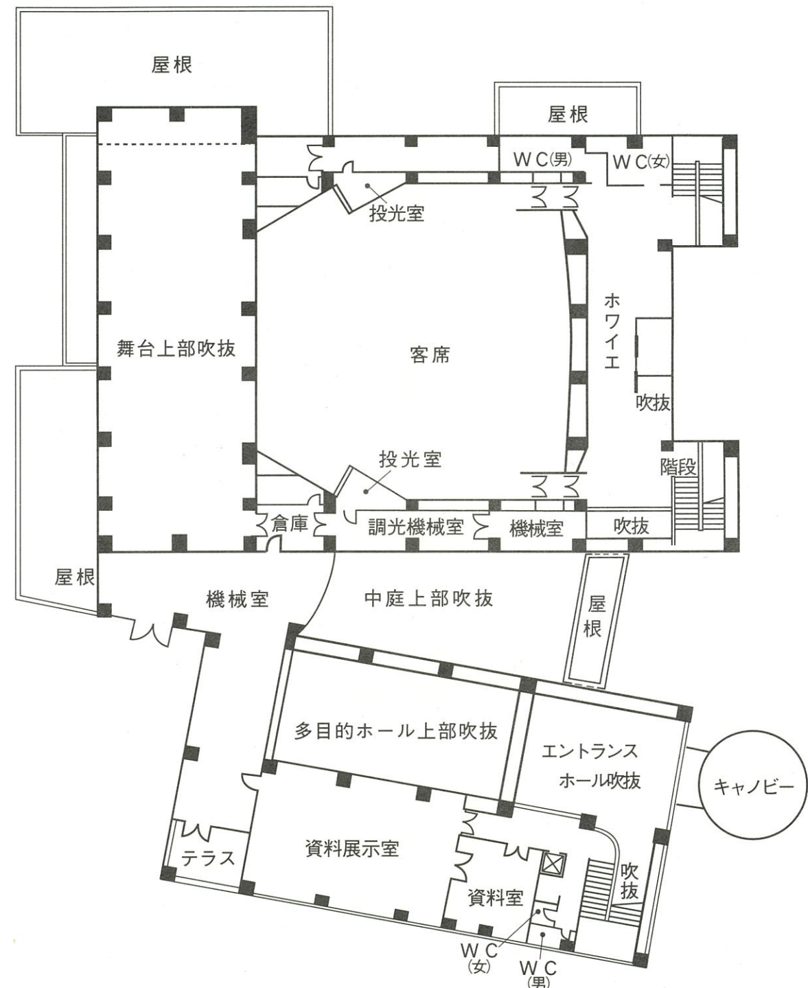
平面図
